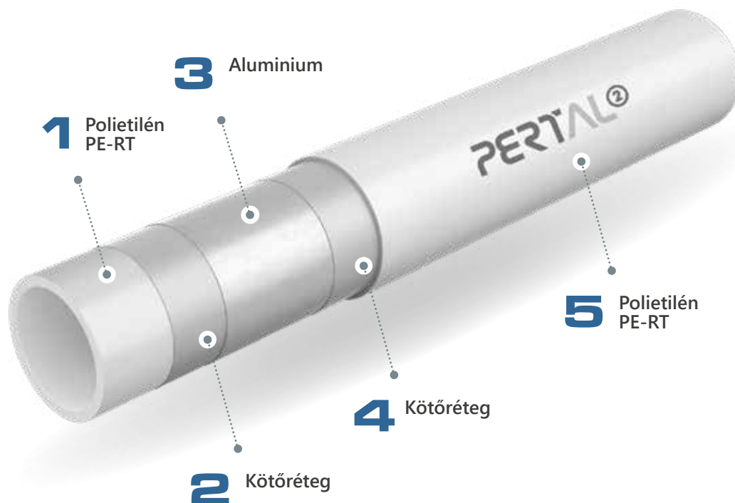
PERTAL 2 cső keresztmetszete
