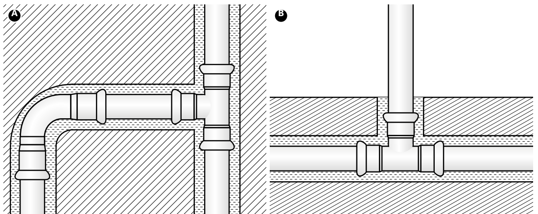
KAN-therm Steel és KAN-therm Inox rendszerek fektetési példák A. falban B. padlóban
