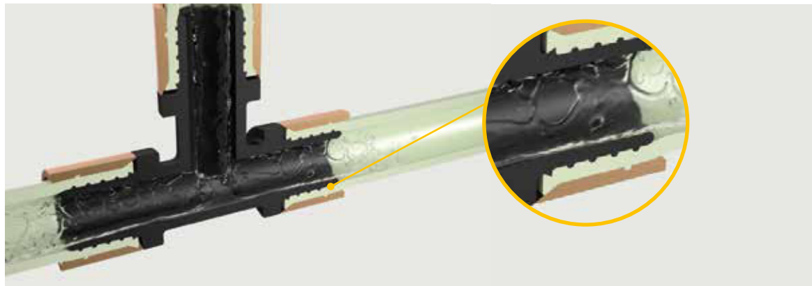
Push kötés keresztmetszete
