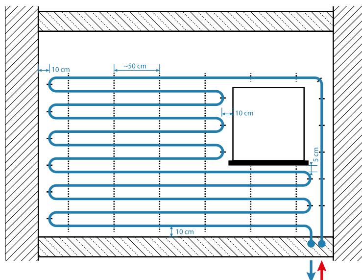
Pic. 34. Szerelési távolságok a falfűtésben.
