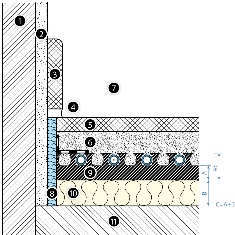
27. Ábra Padlóradiátor KAN-therm Profil rendszerlemezzel és kiegészítő szigeteléssel nem fűtött belső fekvésű helyiségek felett, valamint kültéri levegővel érintkező födémekek felett
