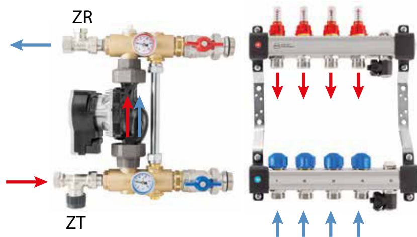
58. Ábra Állandó értékű biztosító szivattyúcsoport UFST elosztóval – áramlási irányok
