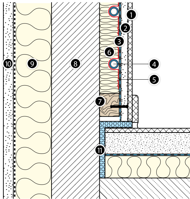
Pic. 36. A KAN-therm TBS falfűtés kiépítése.
