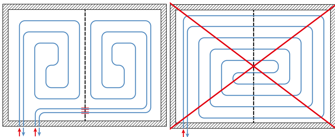
19. Ábra Fűtőmező dilatációs hézaggal megfelelő és nem megfelelő felosztása
