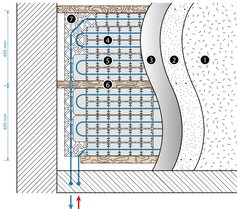
Pic. 37. A KAN-therm TBS falfűtés berendezés keresztmetszete.
