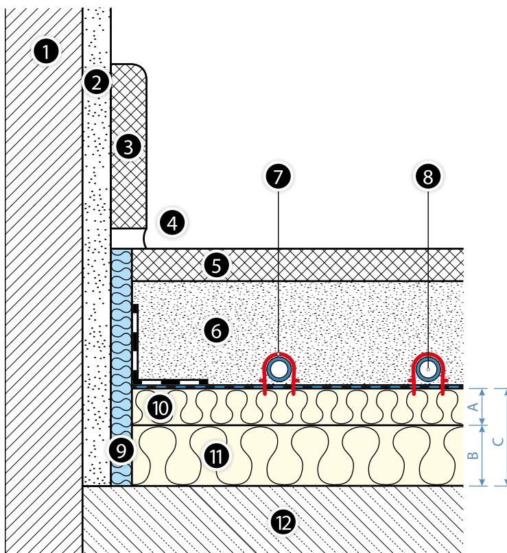
23. Ábra Padlóradiátor rendszerlemezzel és kiegészítő szigeteléssel nem fűtött belső fekvésű helyiségek felett, valamint kültéri levegővel érintkező földmájek felett
