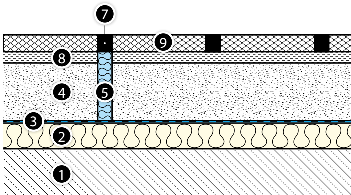
16. Ábra PKőburkolat esetén dilatációs hézag kivitelezése
