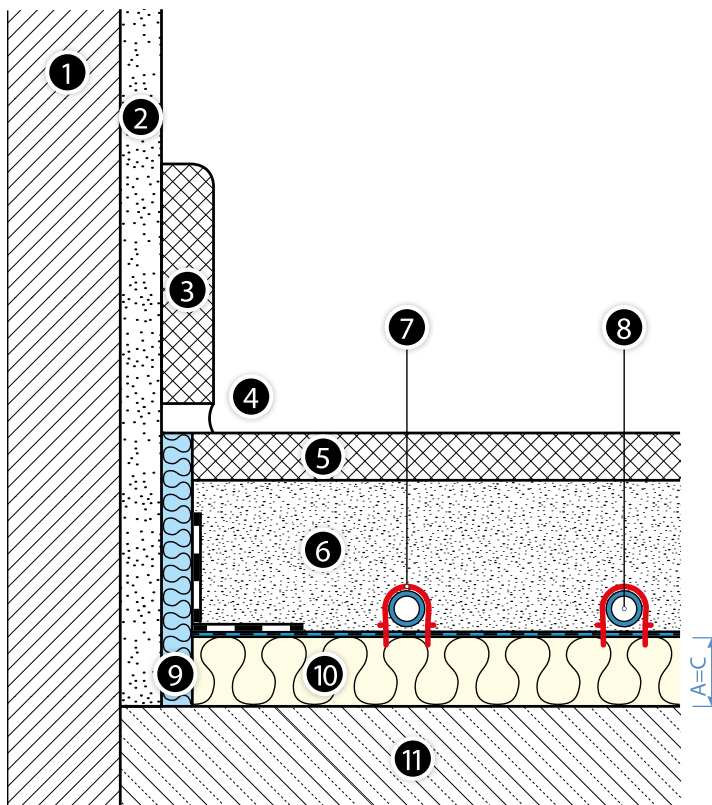
22. Ábra Padlóradiátor rendszerlemezzel belső helyiségek földmáján
