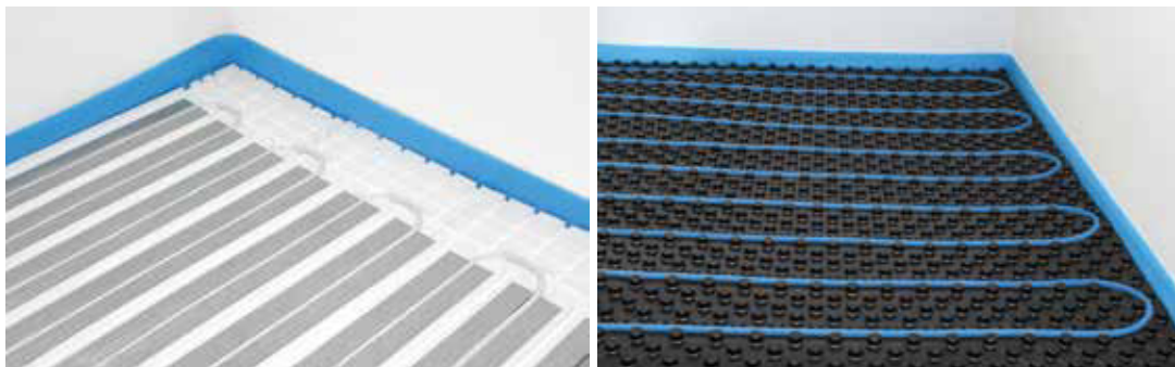
13. Ábra KAN-therm padlófűtés peremszigetelés példák.
