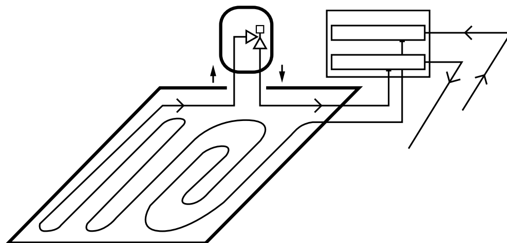
77. Ábra Működési séma – visszatérő ágon elhelyezett berendezés
