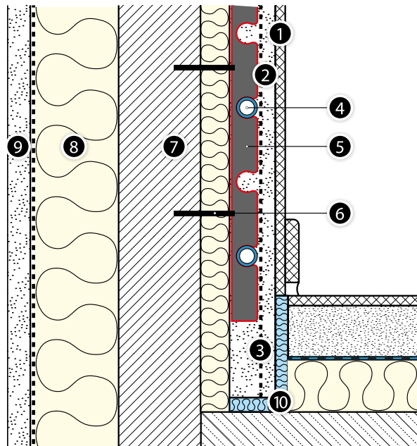
Pic. 35. KAN-therm Rail fűtés telepítése/falhűtés kiépítése.
