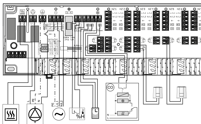
72. Ábra A Basic+ 230 V vagy 24 V terminálblokk műszaki rajza szivattyúmodullal, kazánmodullal és perifériás eszközökkel.
