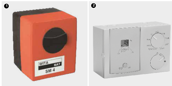
52. Ábra KAN-therm központi keverő rendszer vezérlésének elemei (SM4 (1) működtető és időjáráskövető szabályozó (2))
